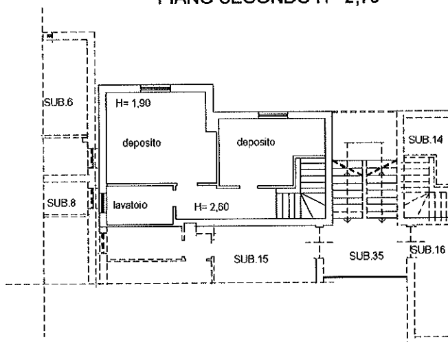
PIANO SECONDO H= 2,70
